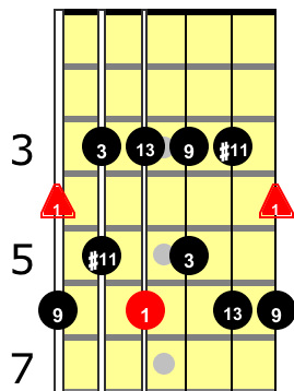
Ab7#11 pentatonic
